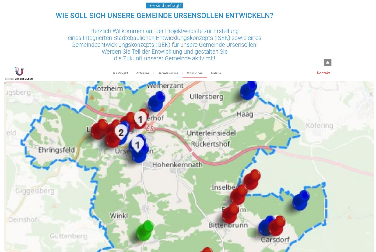
Aufbau Projektwebsite
